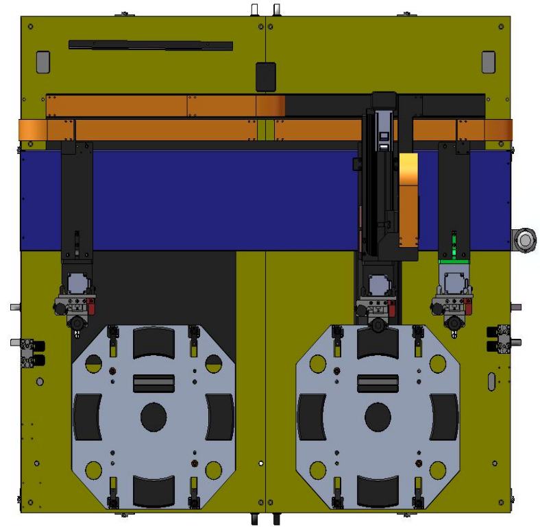
俯视图
