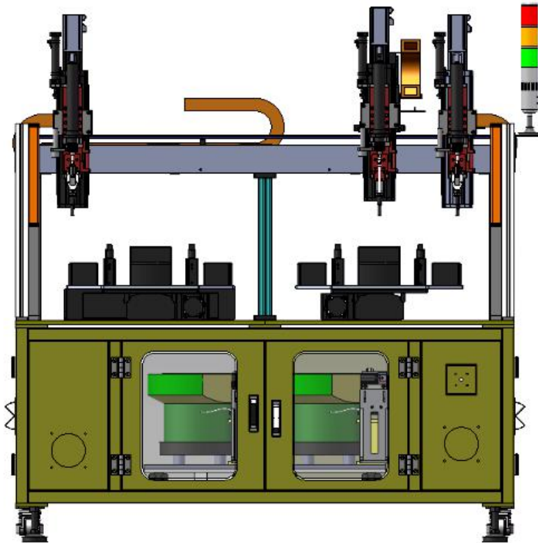
后视图
