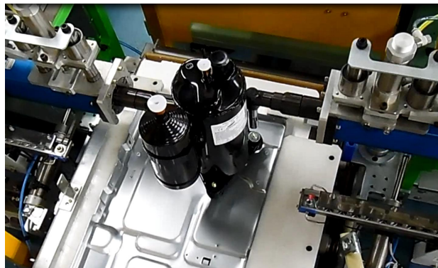
锁付实例
