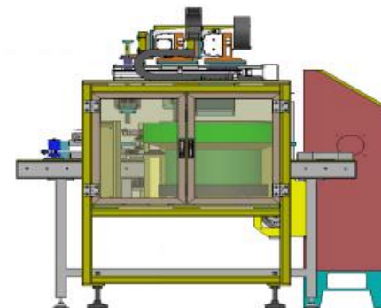
侧视图
