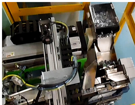
供料单元
