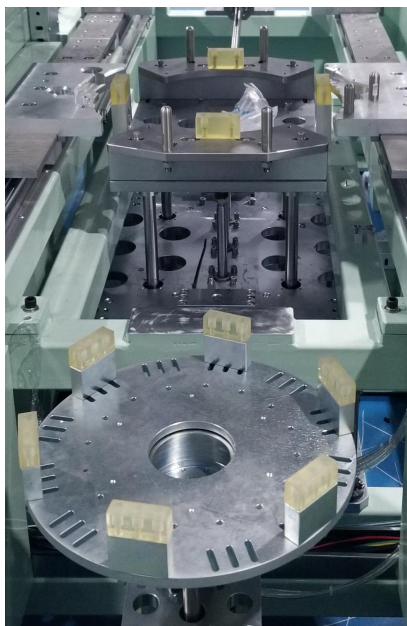
移栽机构
